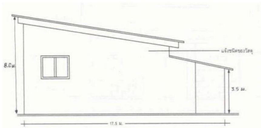
๓. ตัวอย่างแบบแปลนแผนผัง รูปด้านข้าง (ระบุมাত্রาส่วน วัสดุใช้สร้าง)
